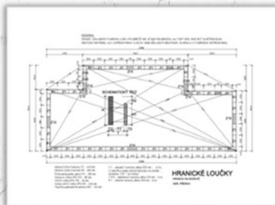
BEZPLATNOU SOUČÁSTÍ KAŽDÉ ZAKÁZKY JE KLADEČSKÝ VÝKRES ULOŽENÍ TVAROVEK
