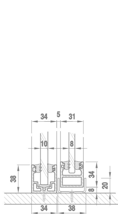
spodní detail
