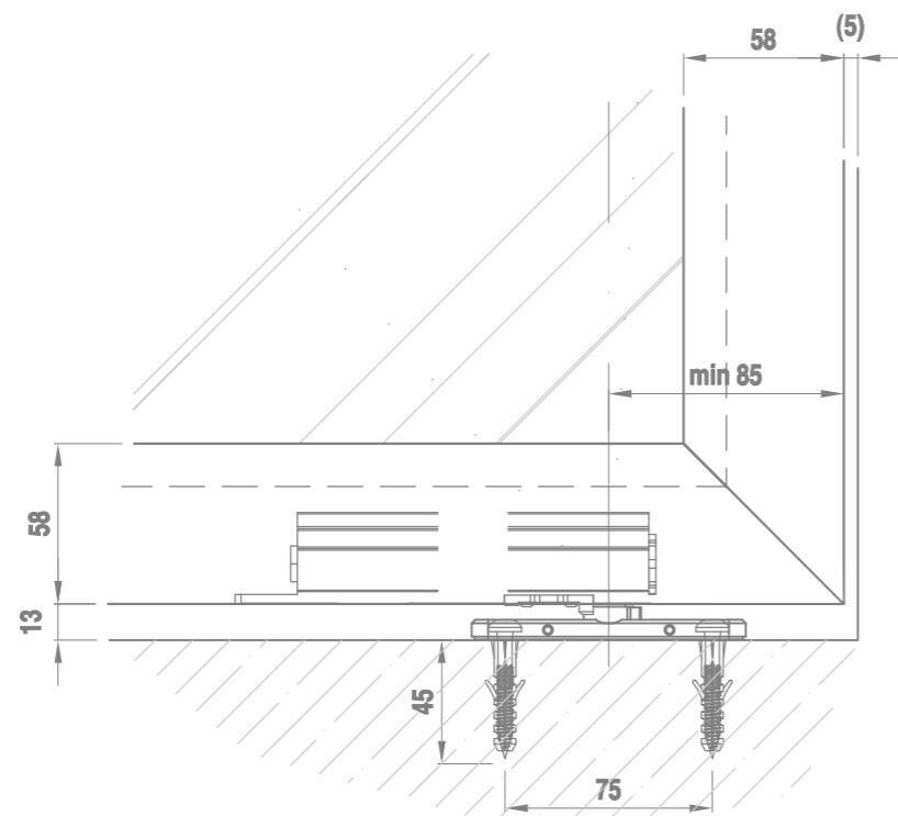
podélný řez - kotvení
