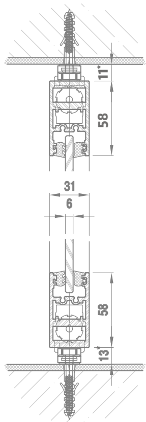
příčný řez - kotvení
