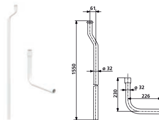
SPLACHOVACÍ TRUBKA S KOLENEM Obj. č. 01 A02 01 0099
