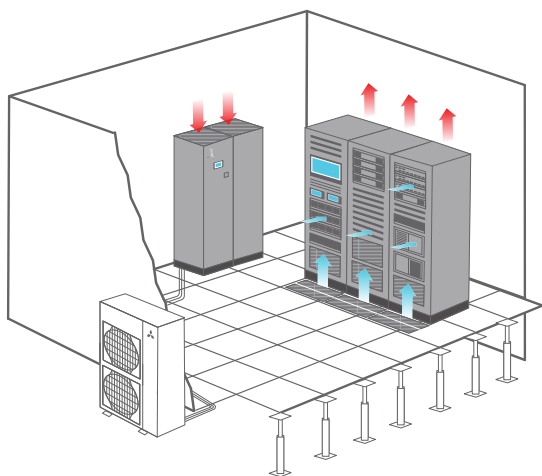
Klimatizační skříň s-MEXT v provedení „Under“ s volitelným ventilačním otvorem pro výstup vzduchu
