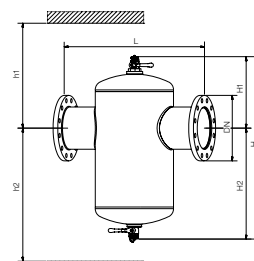
Separátor nečistot
