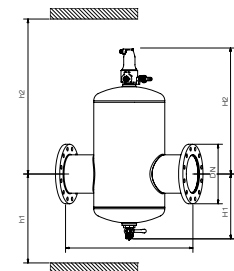
Separátor mikrobublin
