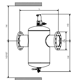
Separátor nečistot
