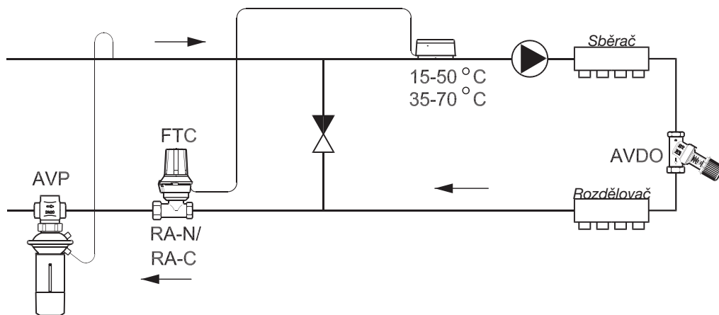
Přímočinná regulace teploty, např. pro podlahové vytápění
